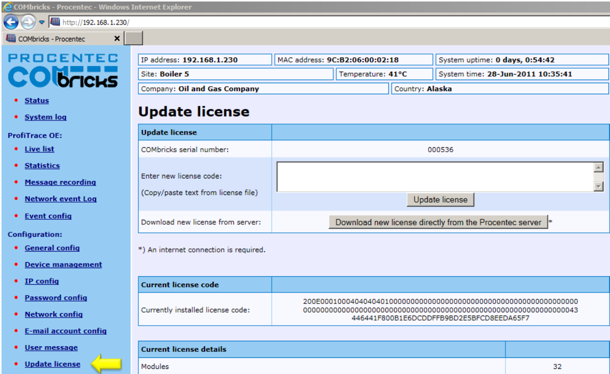
Fig. 37 - License update
