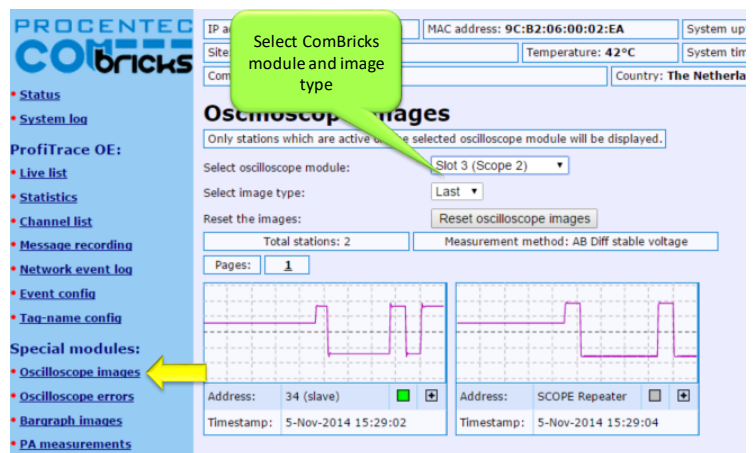
Fig. 49 - Oscilloscope images
